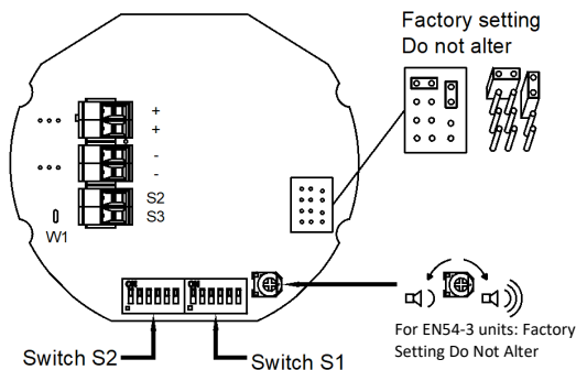
Fig 5: DC PCBA.
