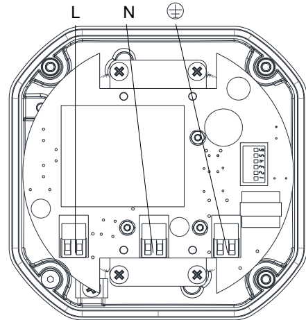
Fig. 3 D2XB1LD2 AC Terminals
