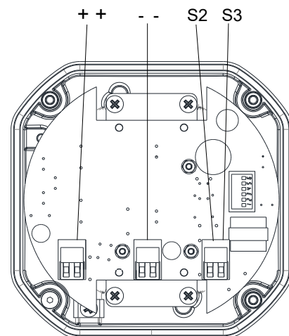
Fig. 4 D2XB1LD2 DC Terminals
